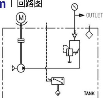
AMGP-013(F), 015(F) Proportional expression / 比例式
