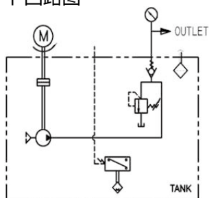
AMGP-01M(F), 01MF-T03 Proportional expression / 比例式
